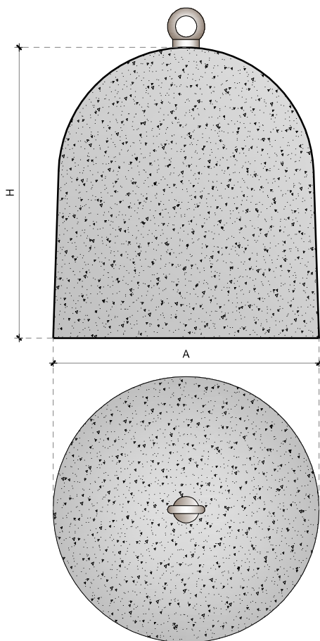
VISTA DALL'ALTO
