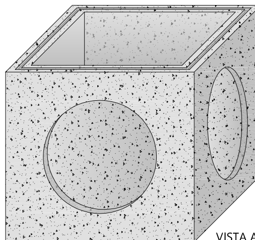
VISTA ASSONOMETRICA
