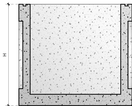
SEZIONE
